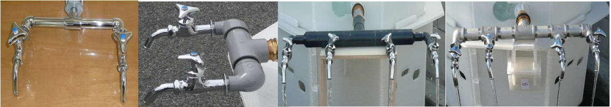
ワンタッチ可能 ・15mm 2口水栓 20mm 2口水栓 20mm 4口水栓 (樹脂製) 20mm 4口水栓
