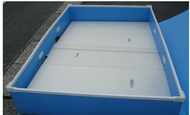
④ 架台、天板収納、パルプ類、受台、充填口固定柵を収納
